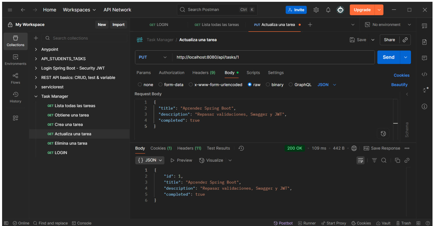
Prueba de Endpoint PUT para: Actualizar una tarea
