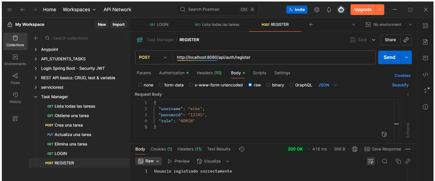
Prueba de Endpoint POST para: Crear un usuario ADMIN
