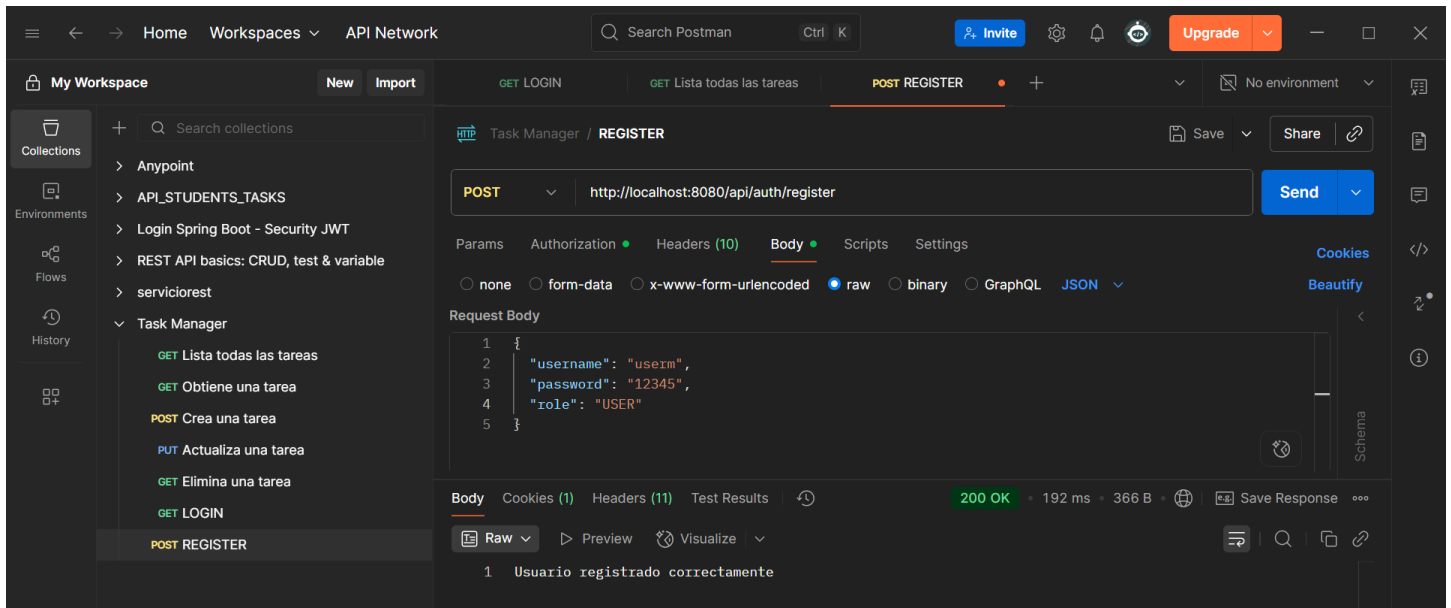
Prueba de Endpoint POST para: Crear un usuario normal
