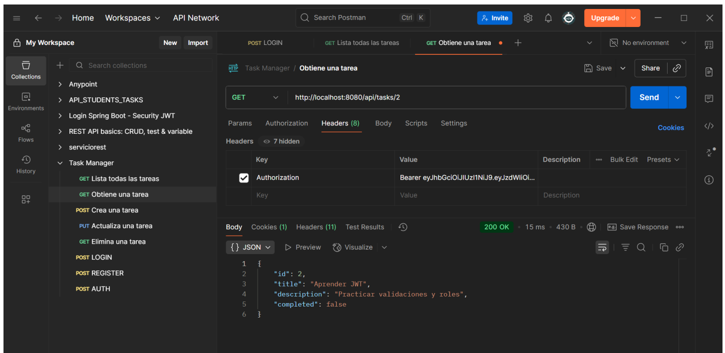
Prueba de Endpoint GET para: Obtener una tarea mediante su ID
